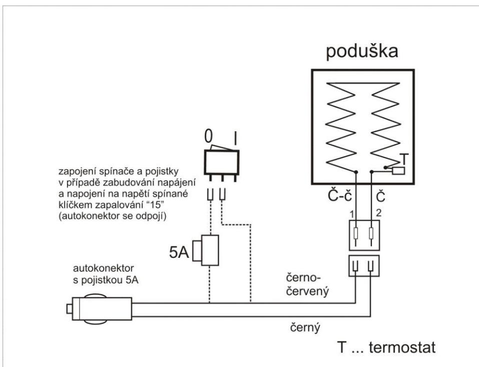
Obr. Schéma elektrického vyhřívání sedadla HTS – 101
